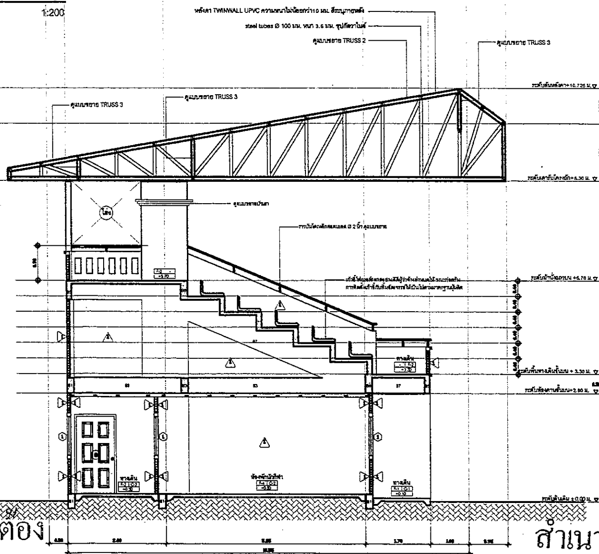
รูปตัด B-B
