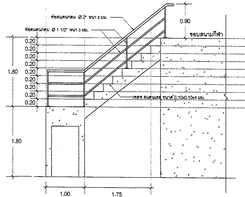
แบบขยาย รวบบันได 2 SCALE 1:50
