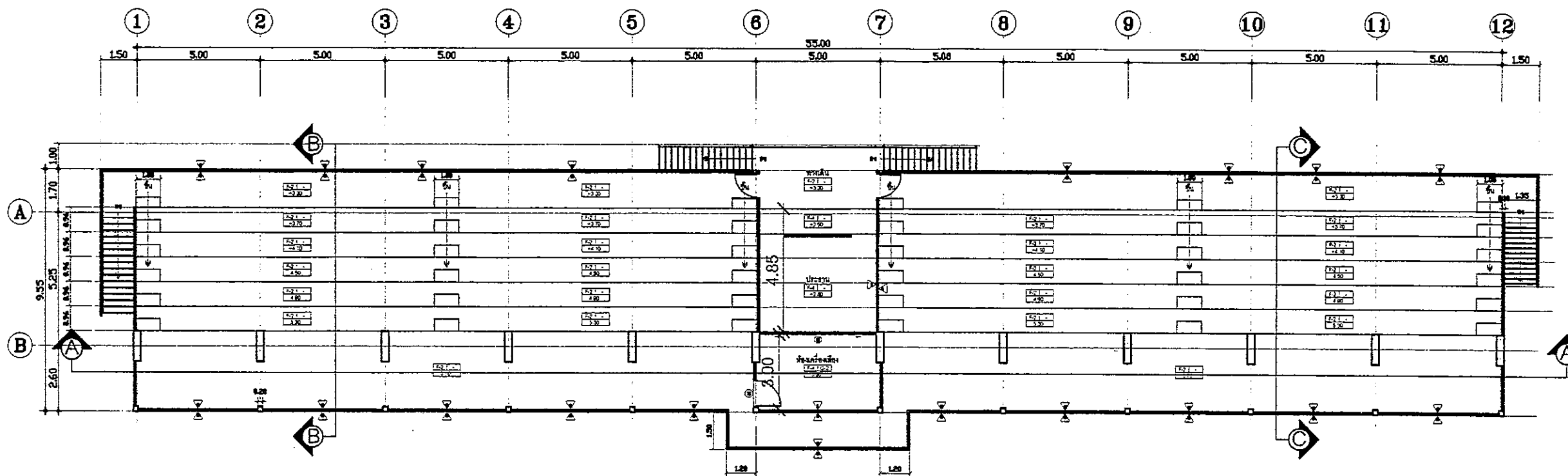
แปลนพื้นชั้นจันทน์ SCALE 1:200
