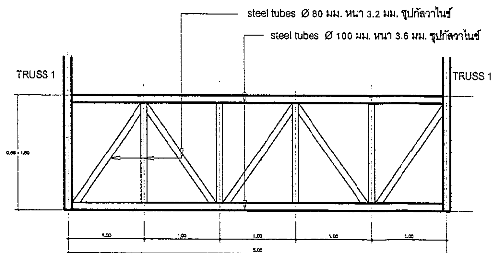
แบบขยาย TRUSS 3 SCALE 1:50
