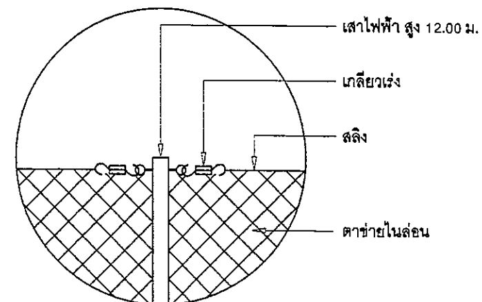
แบบขยาย SCALE 1:100
