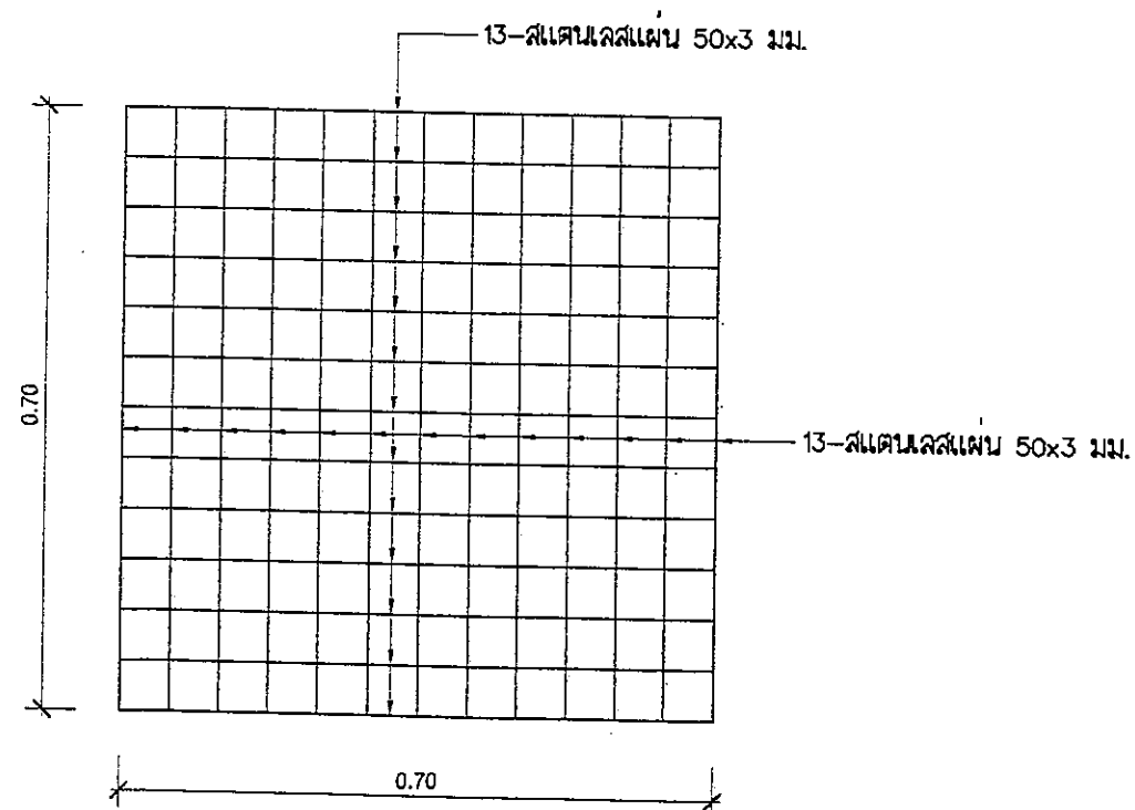
แบบขยายฝาบ่อพักตะแกรงสแตนเลส SCALE 1:10
