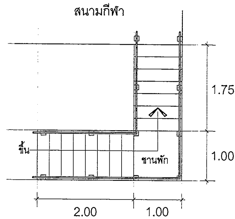
แปลนพื้น รวบบันได SCALE 1:50
