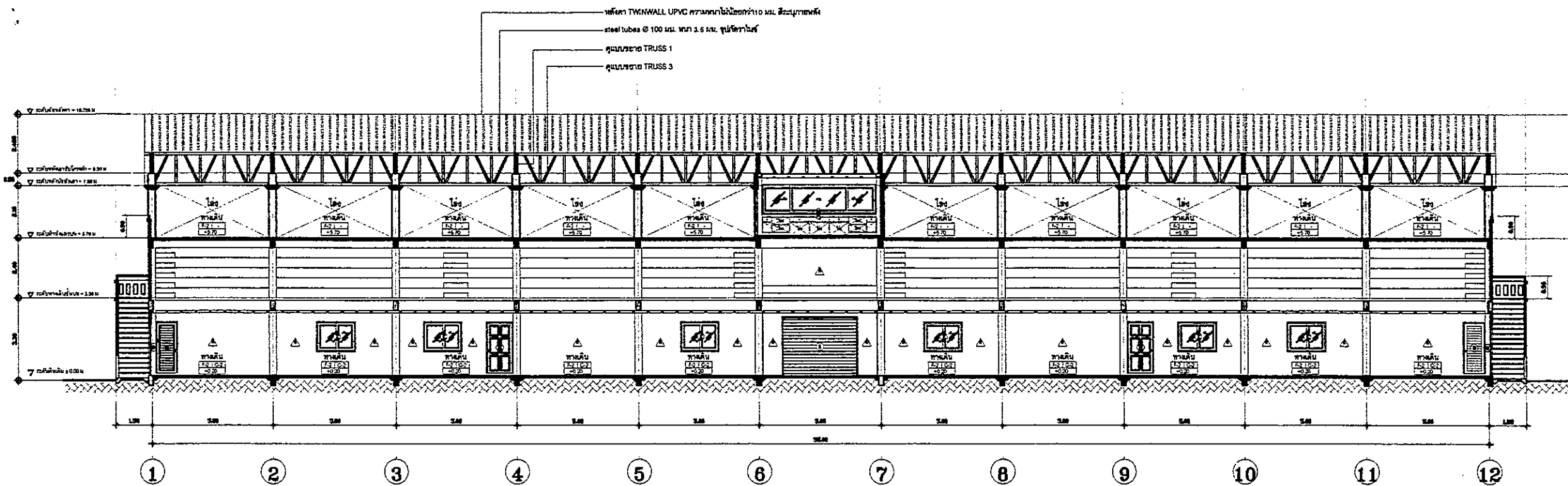
รูปตัด A-A
