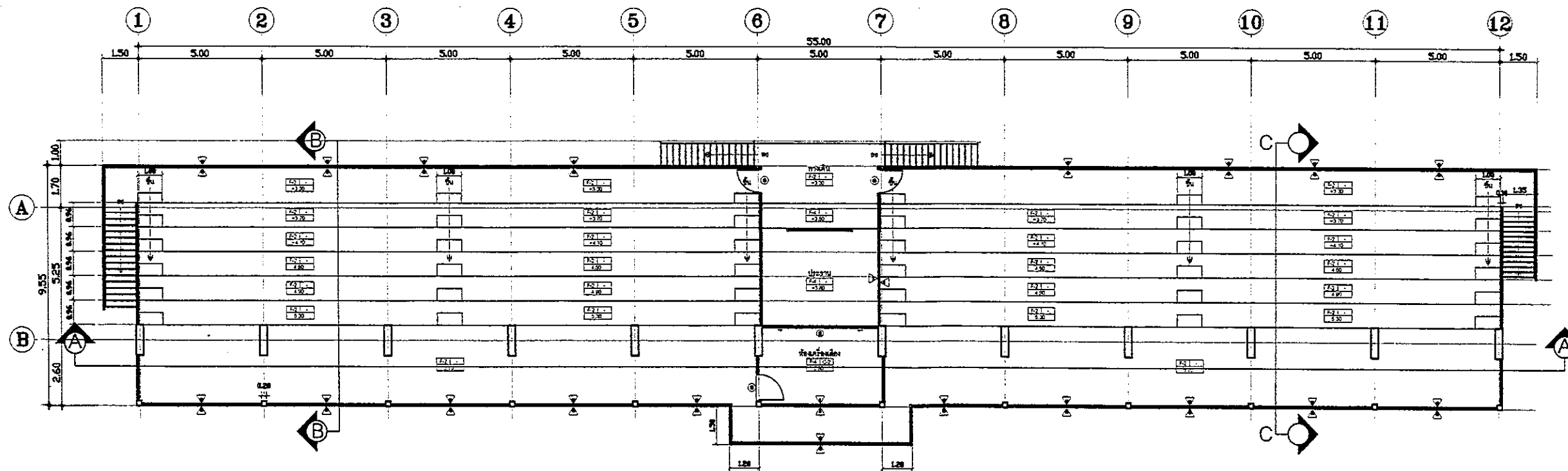
แปลนพื้นชั้น 2 SCALE 1:200
