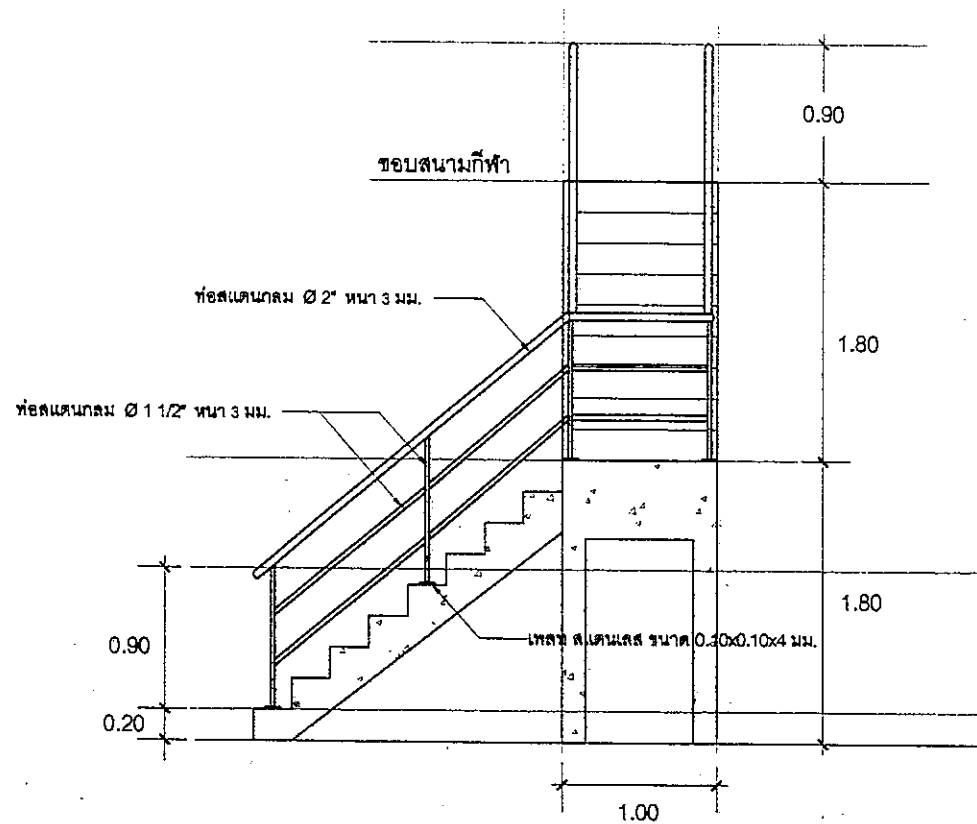
แบบขยาย รวบบันได 1 SCALE 1:50
