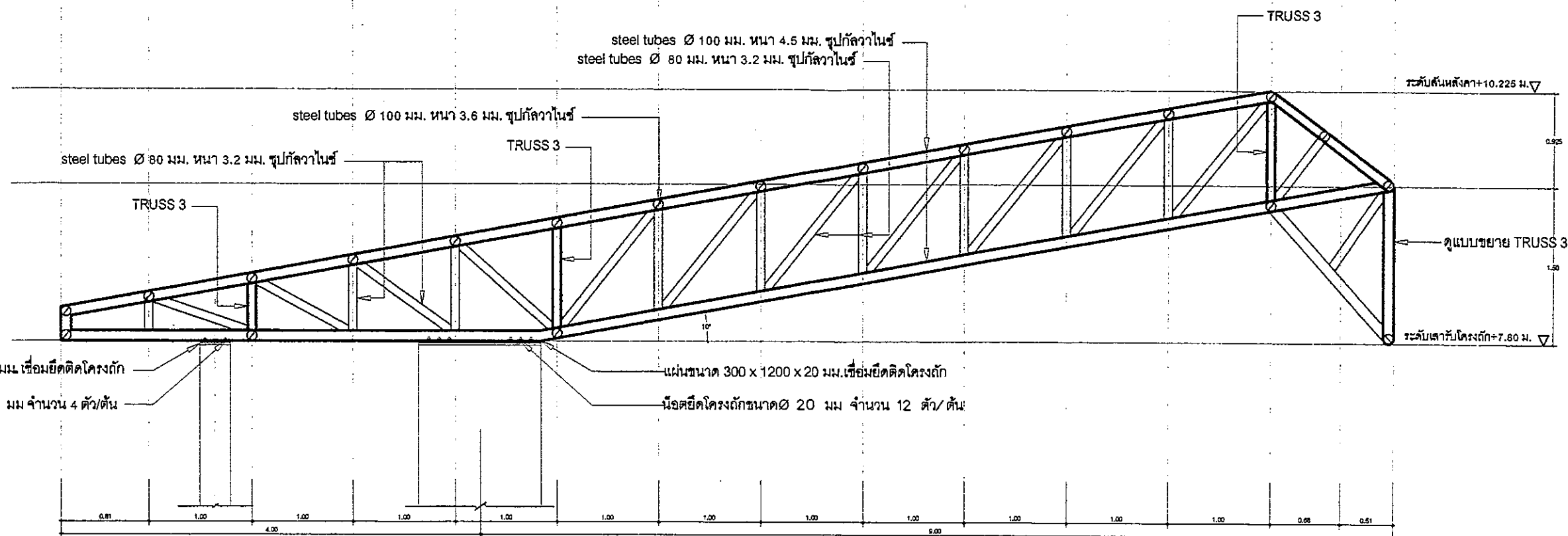
แบบขยาย TRUSS 2 SCALE 1:50
