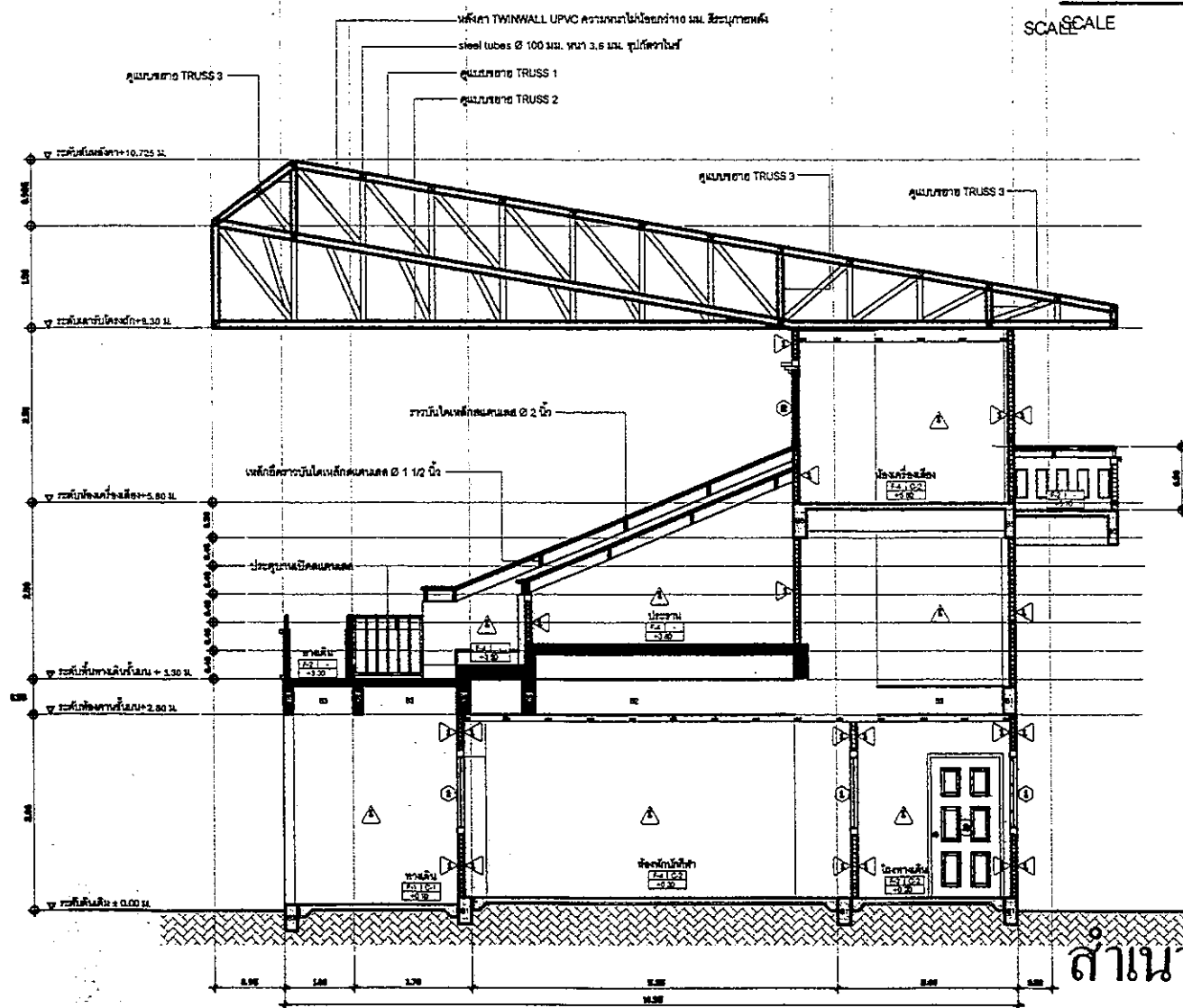
รูปตัด C-C
