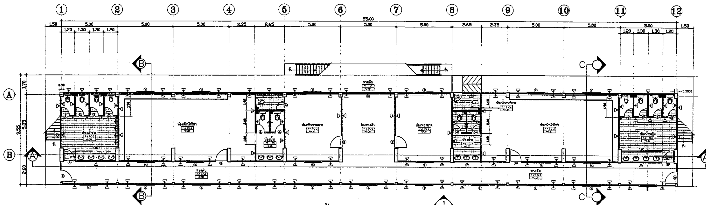
แปลนพื้นห้องใต้ถมจันทร์ SCALE 1:200
